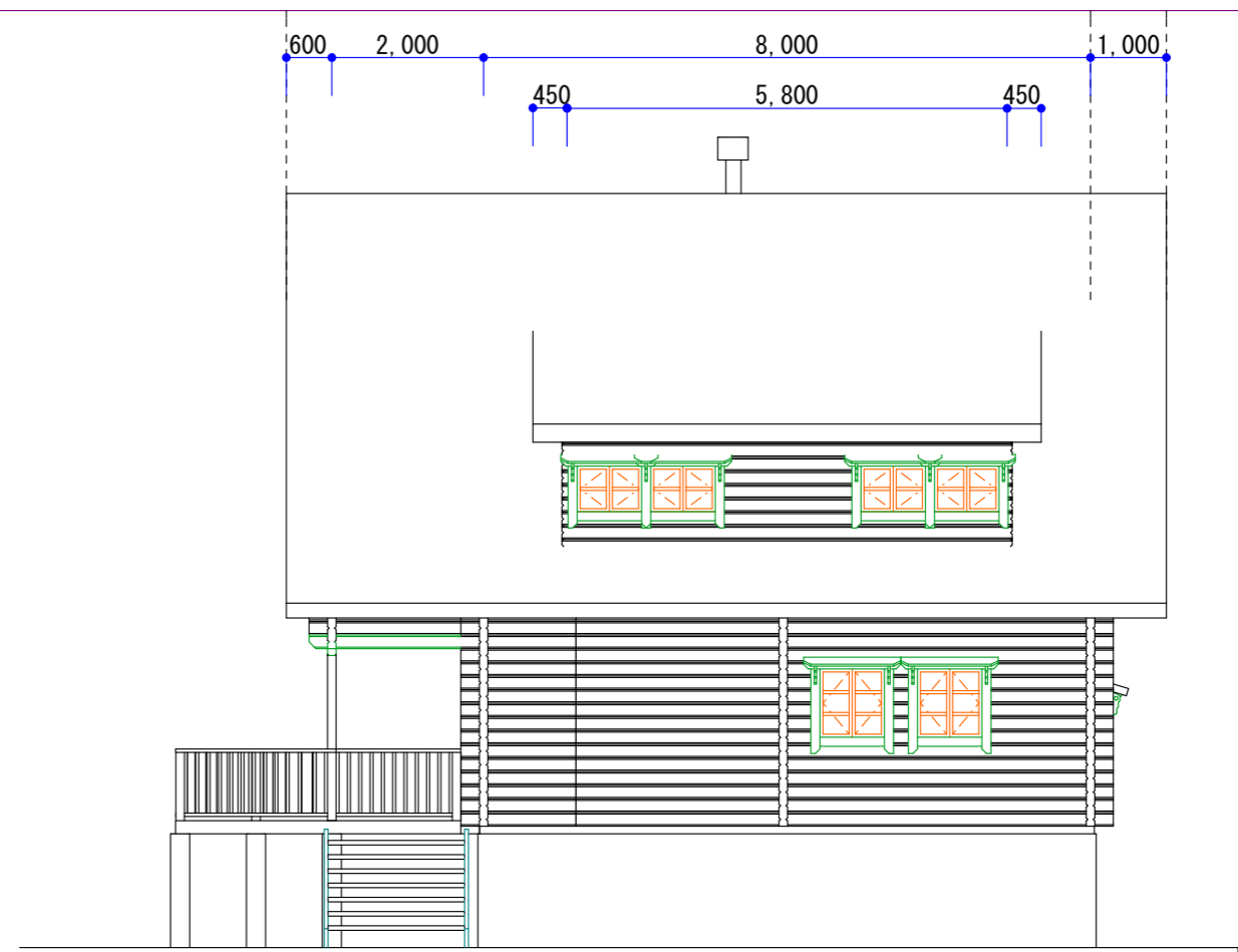
東面 立面図 1:100
