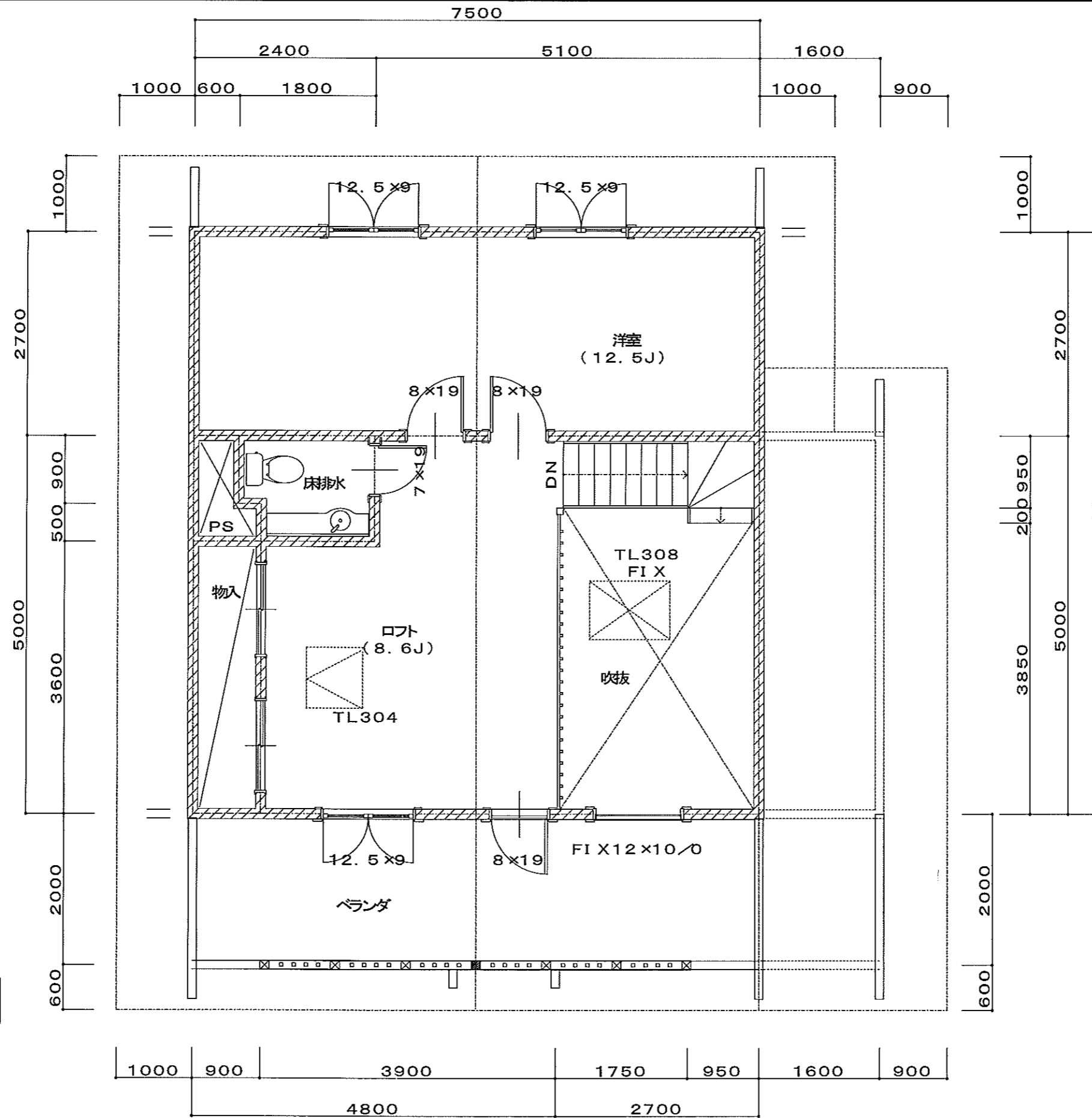
2階平面図 S: 1/60
